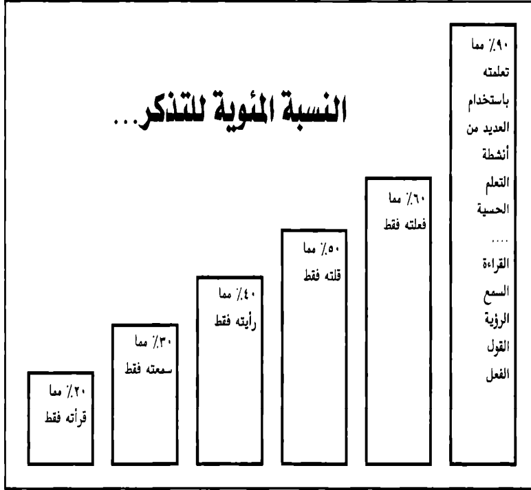
الشكل رقم ٣ الرسم البياني للتذكر
